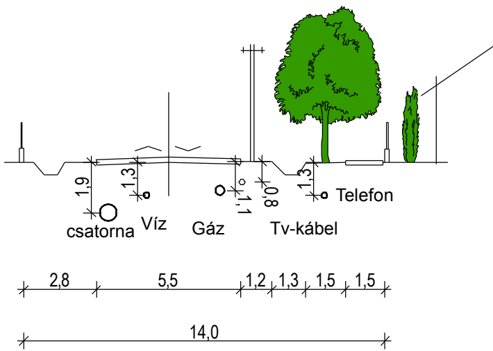
14 m. széles utcák mintakeresztmetszete
