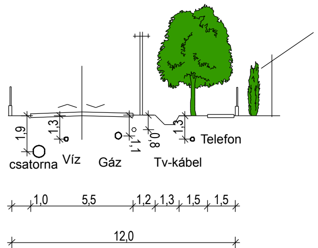
12 m. széles utcák mintakeresztmetszete
